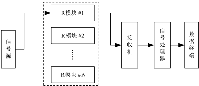
图 16 有源相控阵天线接收机动态范围测试示意图
