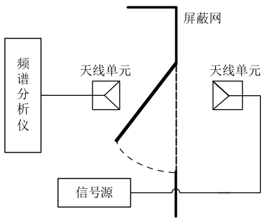
图 6 双程屏蔽网隔离度测试示意图
